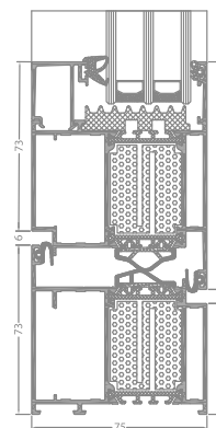
przekrój przez drzwi GN 75 (GN 414 + GN 425)
