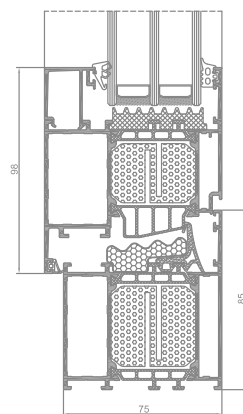
przekrój przez okno GN 75 (GN 013 + GN 022)
